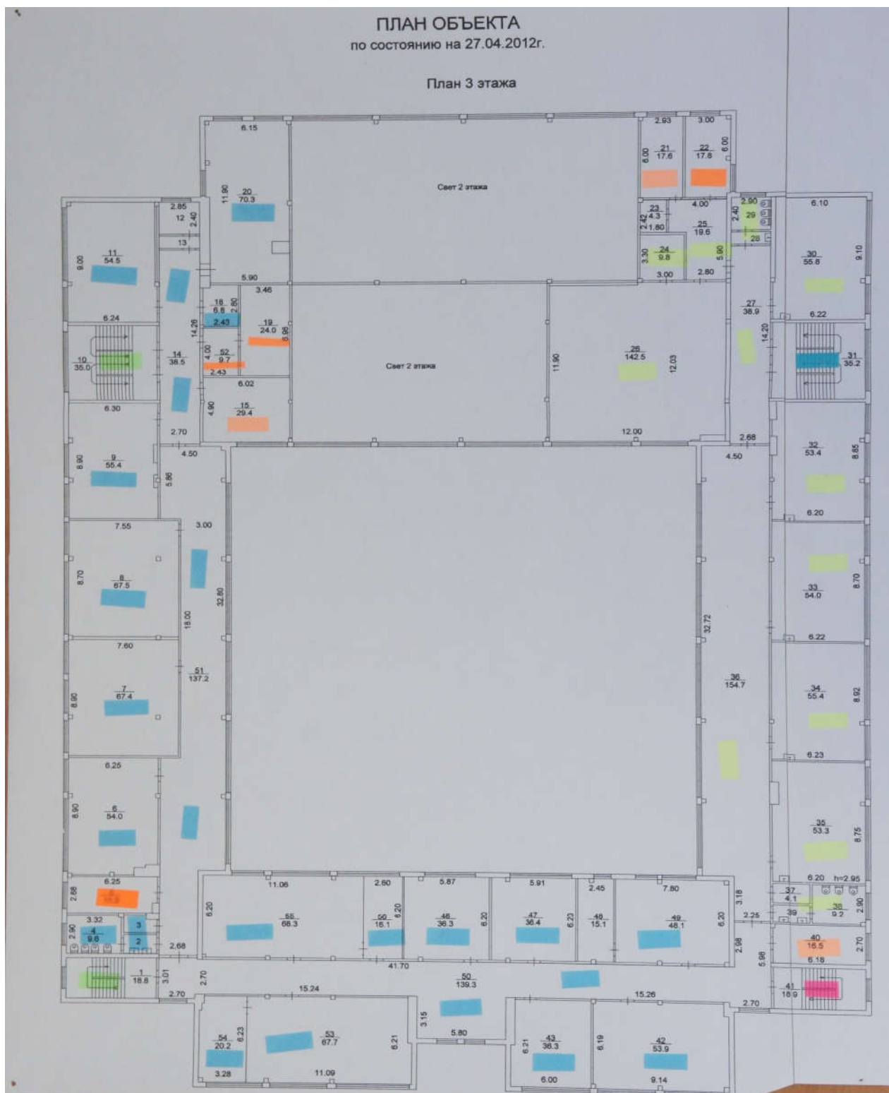
Рис. № 4. План объекта (3 этаж) по состоянию на 27.04.2012 года.
