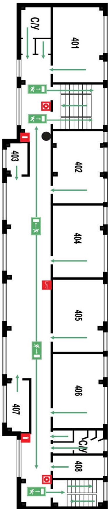
Рис. 20. План эвакуации при пожаре и других ЧС из помещений 4 этажа учреждения.
