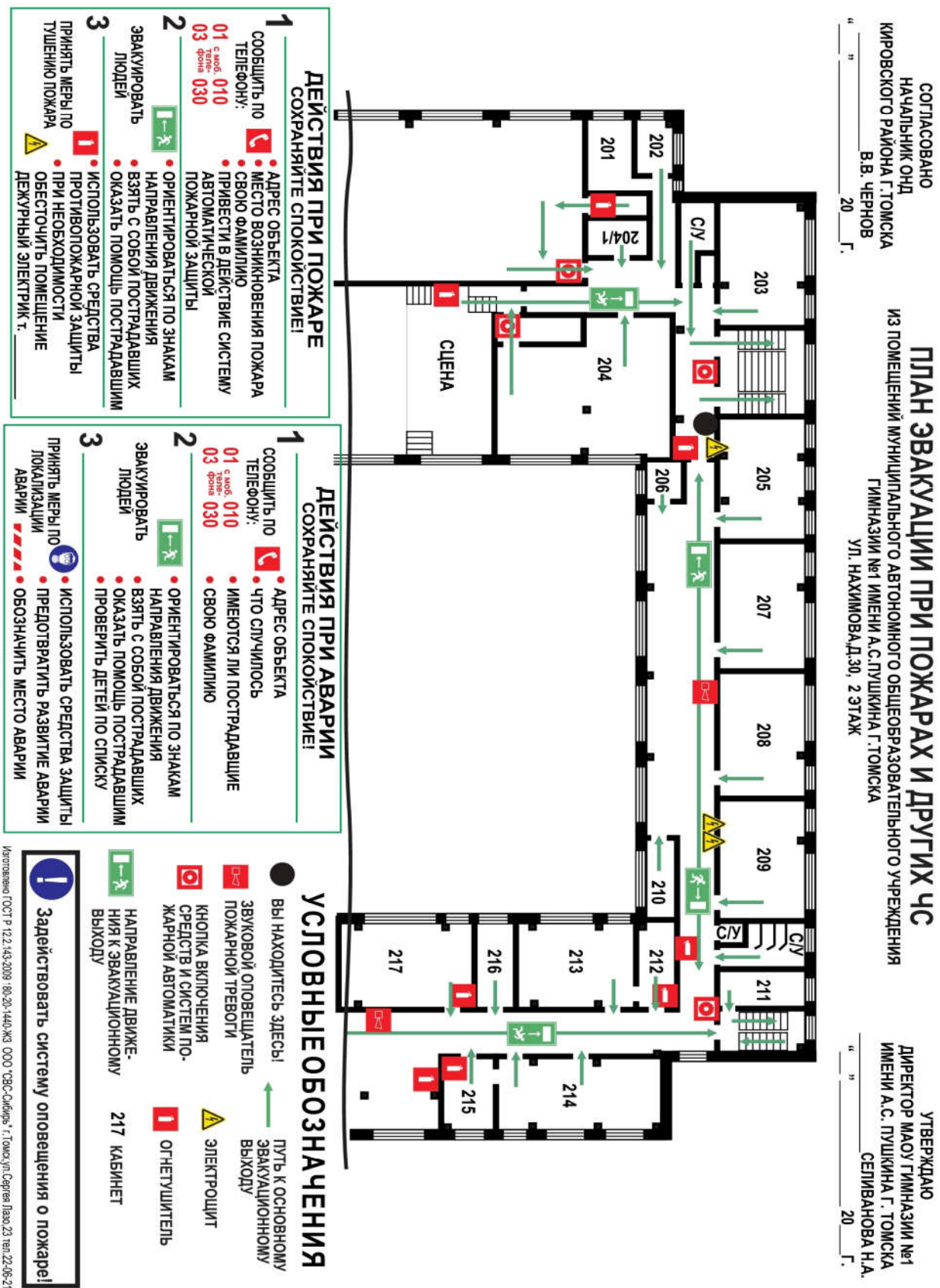
Рис. 17. План эвакуации при пожаре и других ЧС из помещений 2 этажа учреждения.
